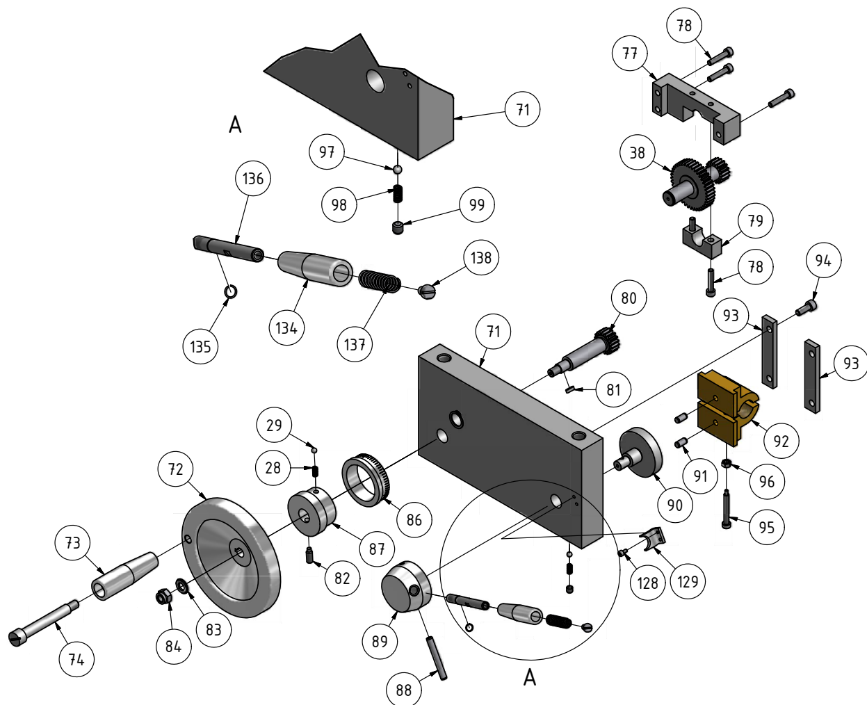
2-3: lathe saddle D280
