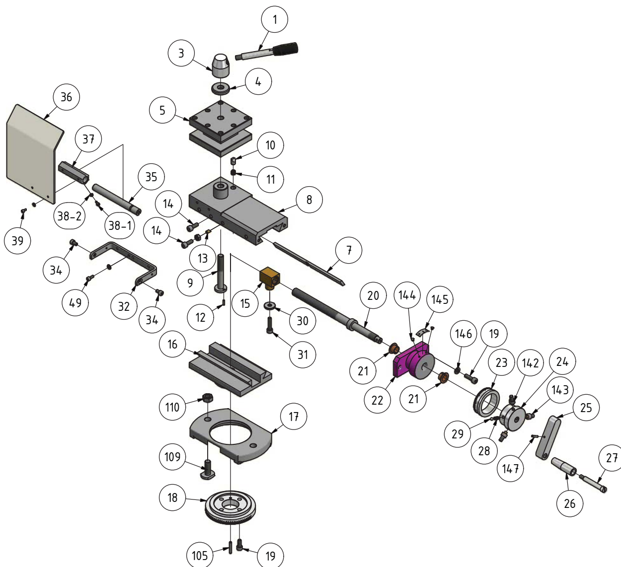
2-1: Top slide D280
