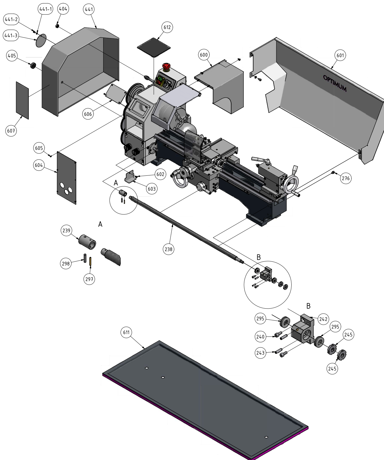
1-6: Machine bed D240
