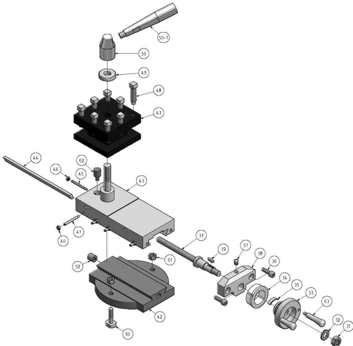
Abb.6-1: Oberschlitten - Top slide
