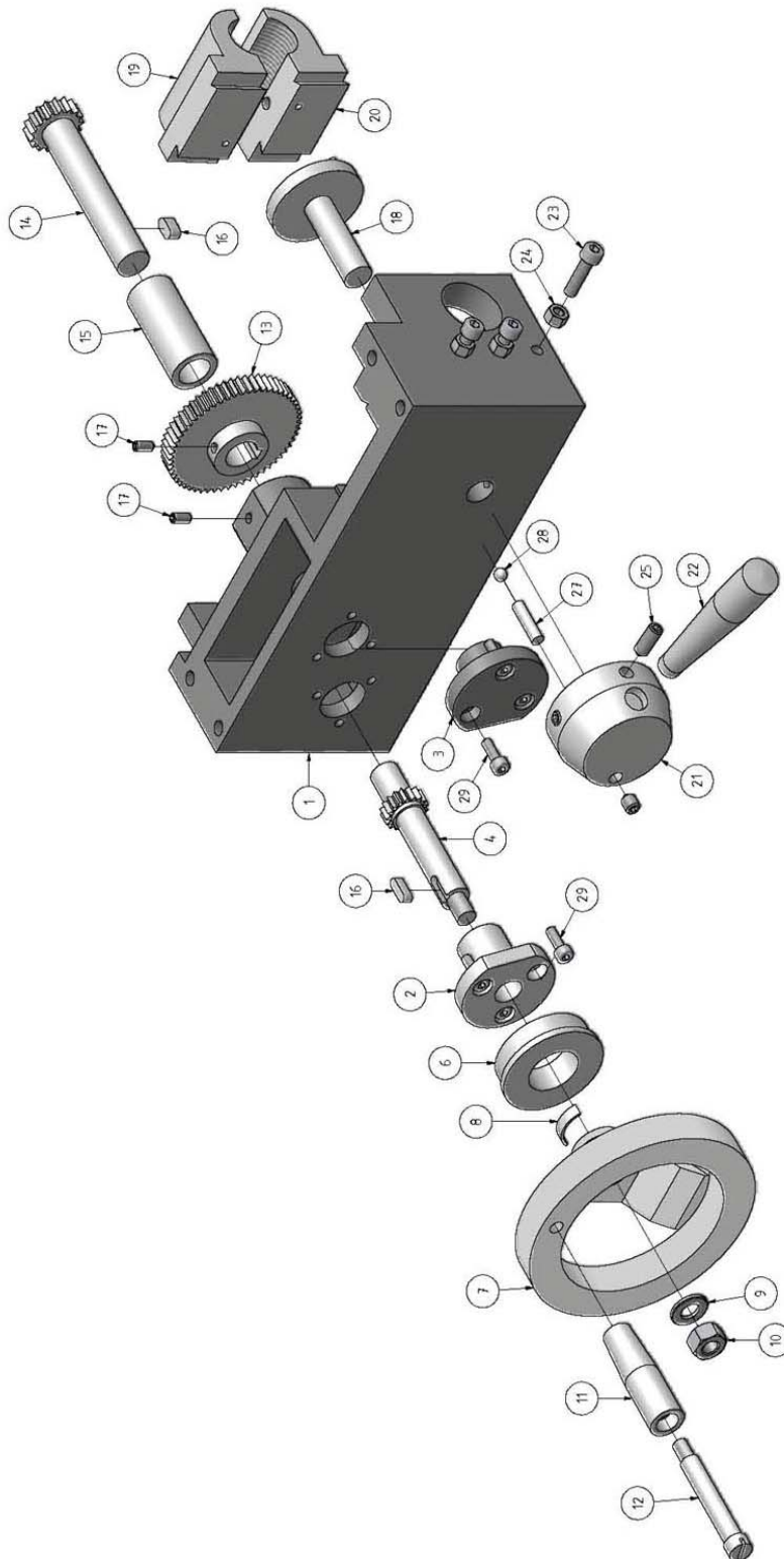
Abb. 6-4: Bettschlitten - Bed slide
