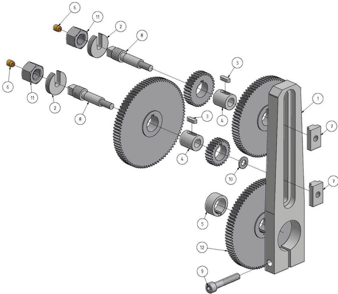
Abb.6-3: Wechselradschere
