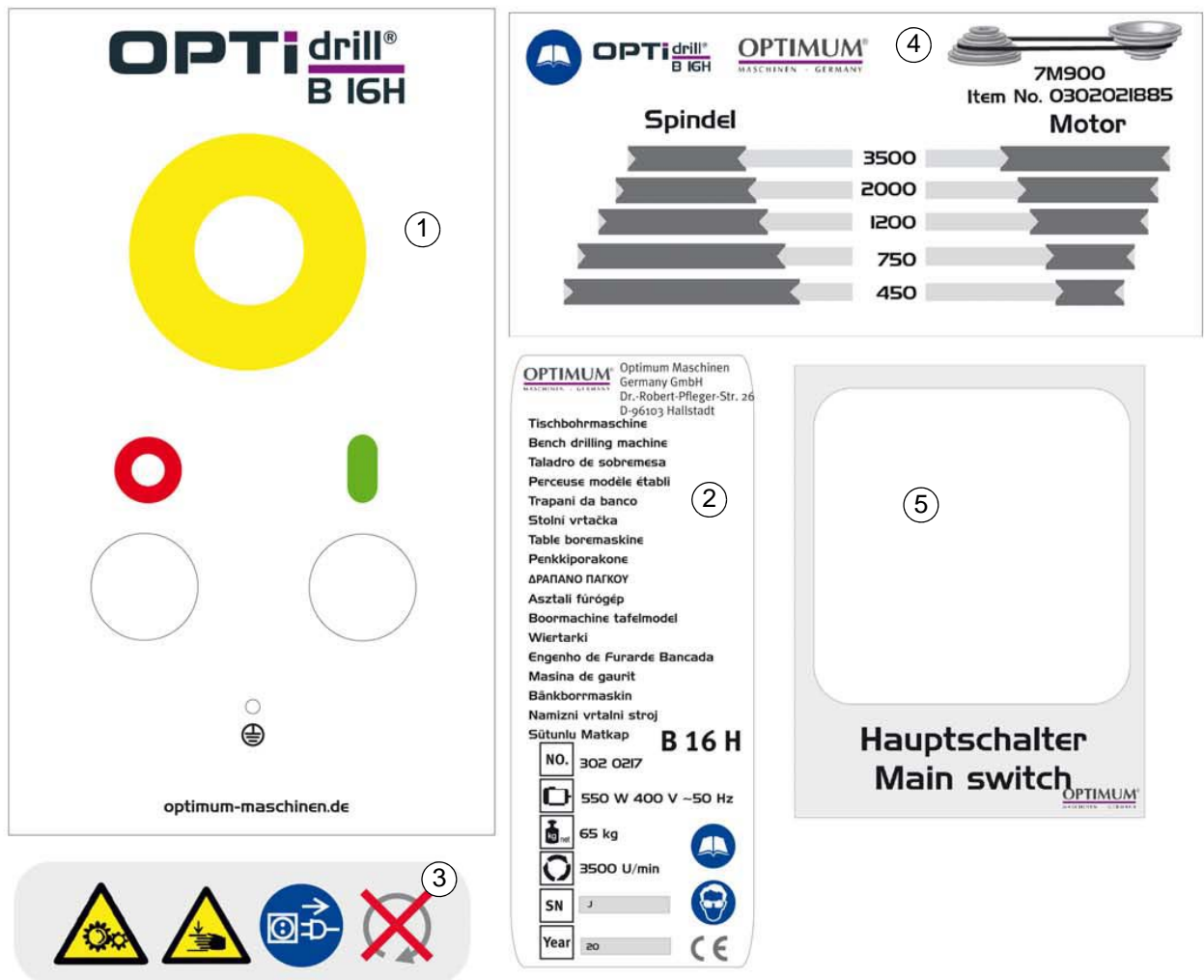
Abb. 7-1: Maschinenschilder - Machine labels
