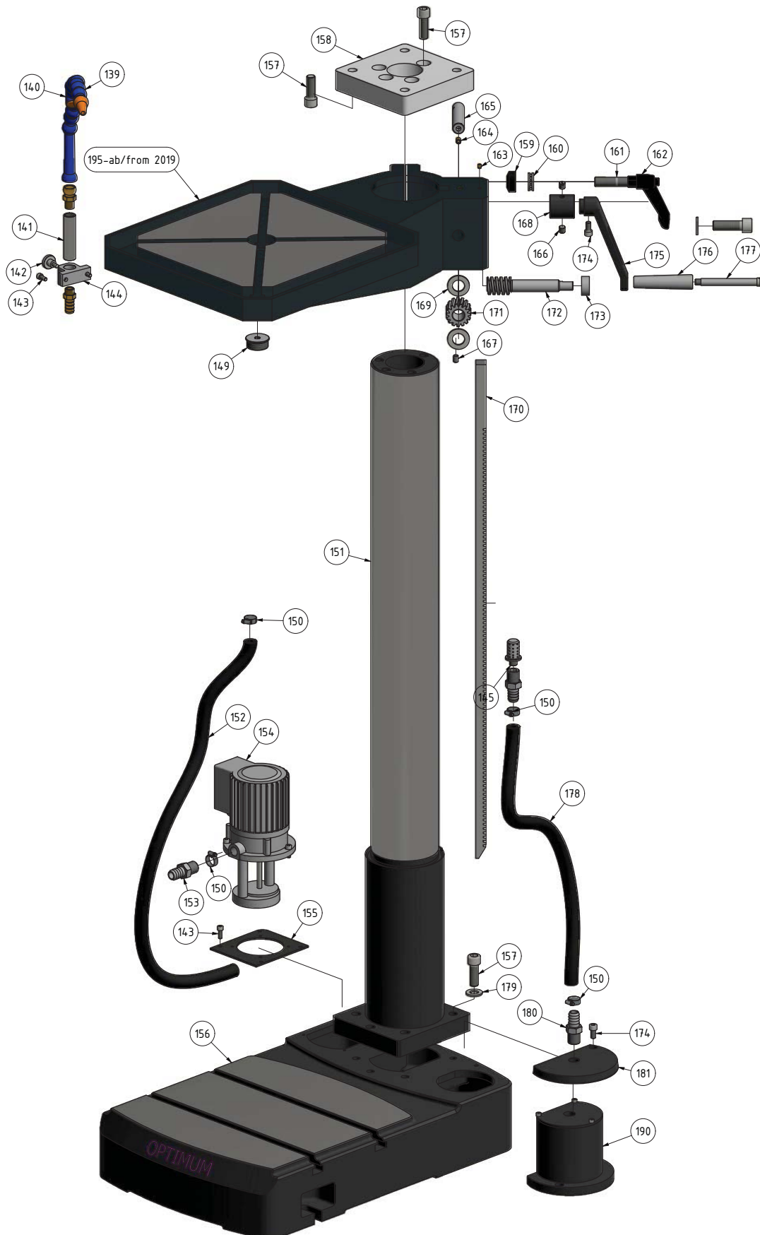
Abb.1-18: Säule und Bohrtisch - Column and drilling table
