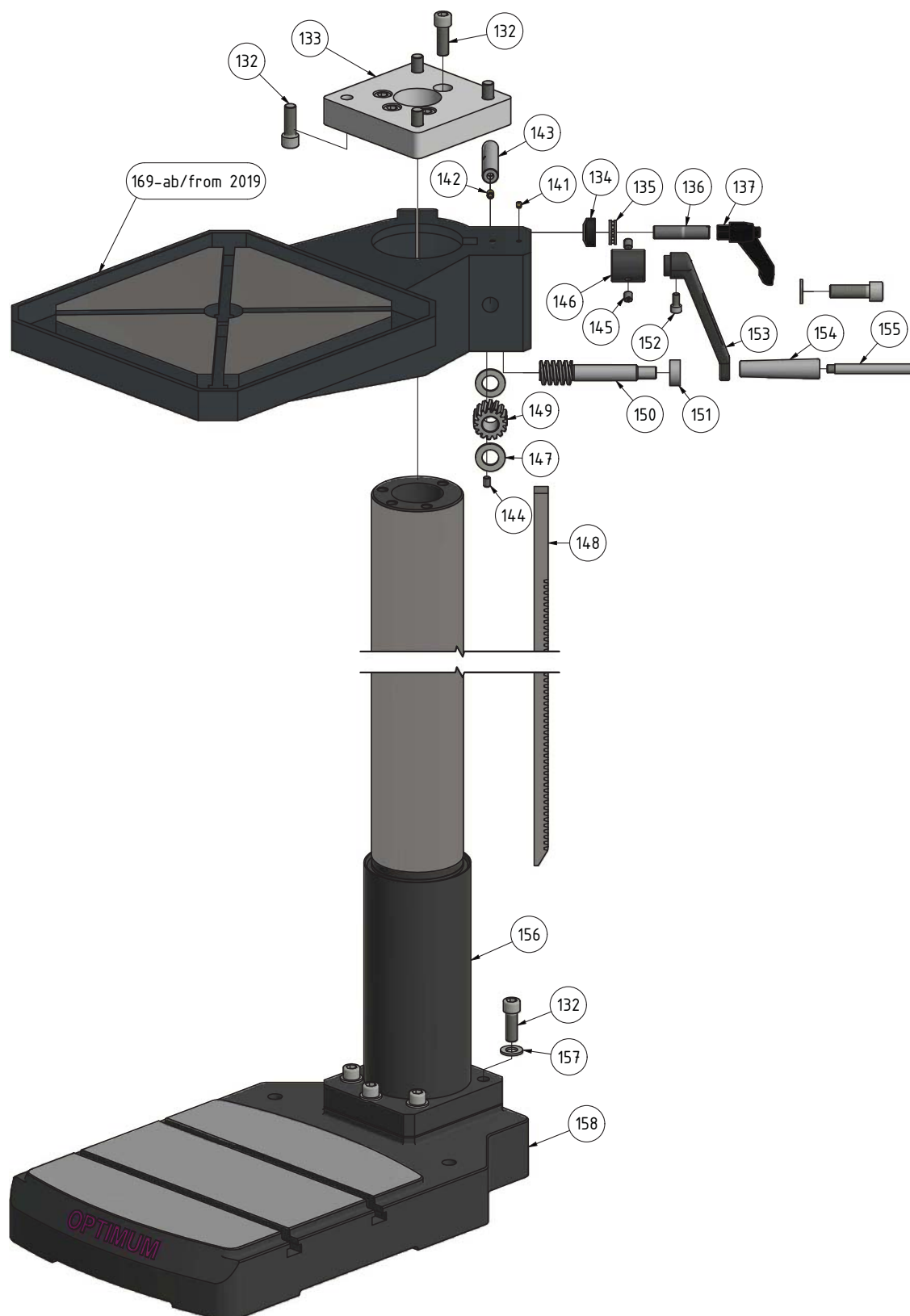
Abb.1-8: Säule und Bohrtisch - Column and drilling table
