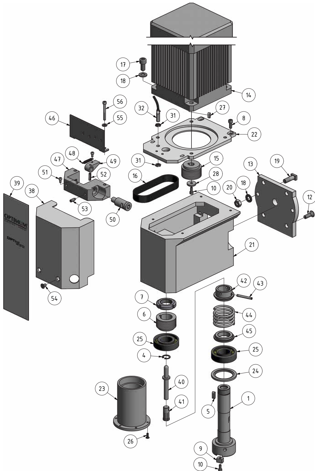
Img.1-1: Fräskopf - Milling head
