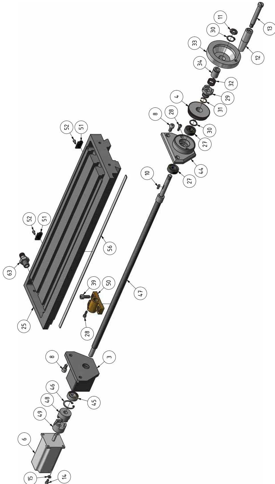
Img.1-5: Frästisch - Milling table 2-2
