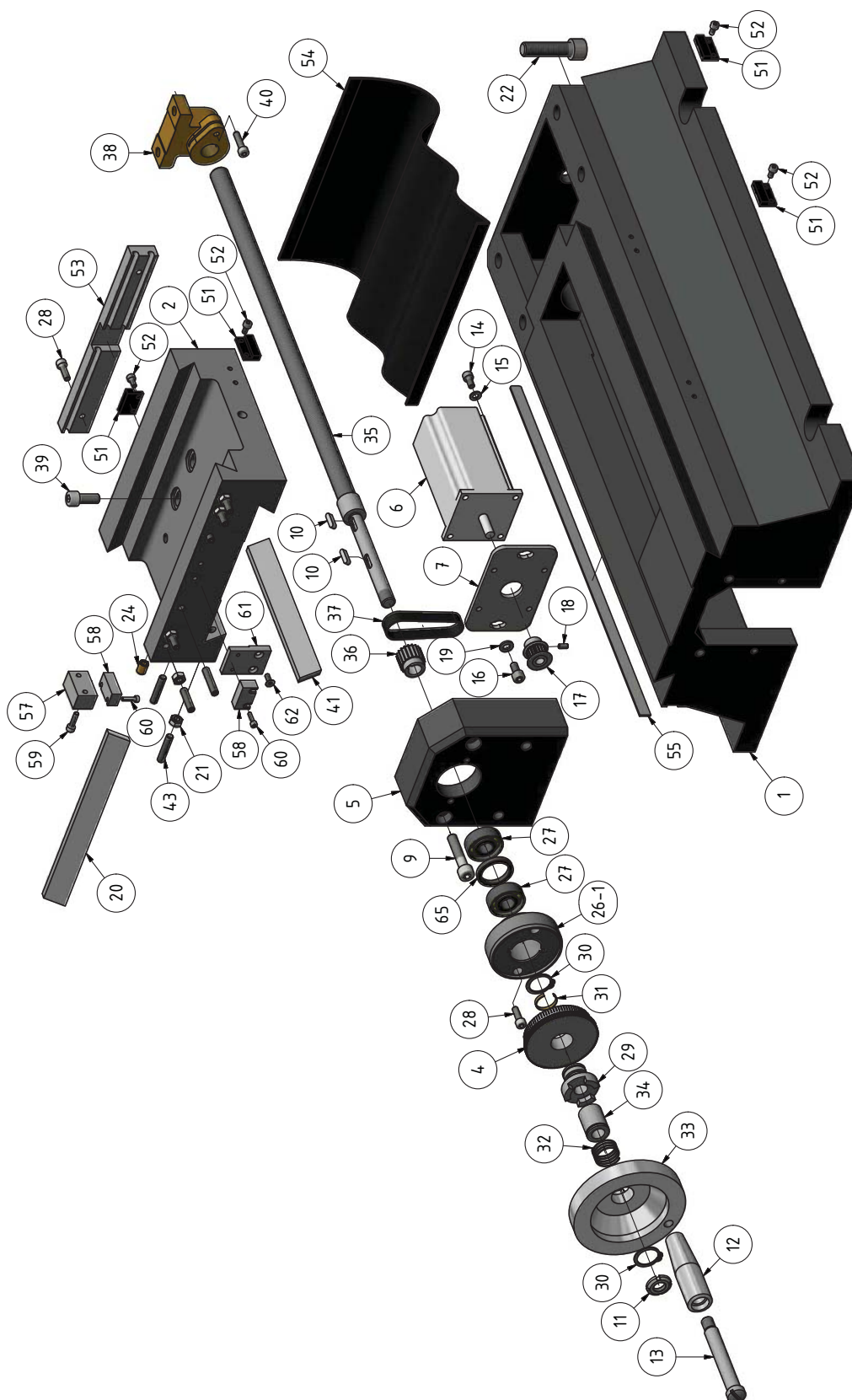
Img.1-4: Frästisch - Milling table 1-2
