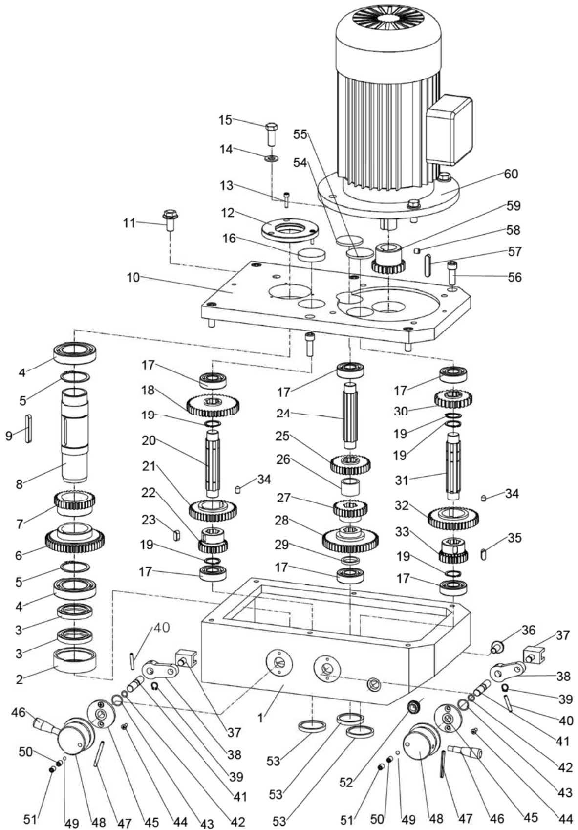
Abb.1-3: Schaltgetriebe Vertikalfräsen - Transmission gear vertical milling
