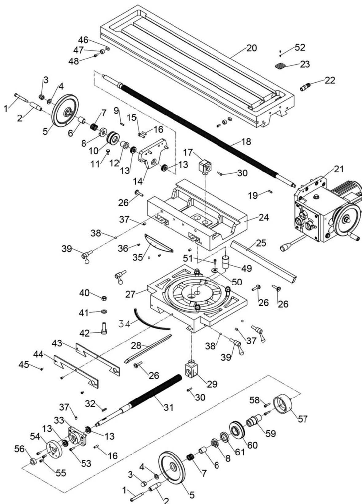
Abb.1-2: Frästisch - Milling table
