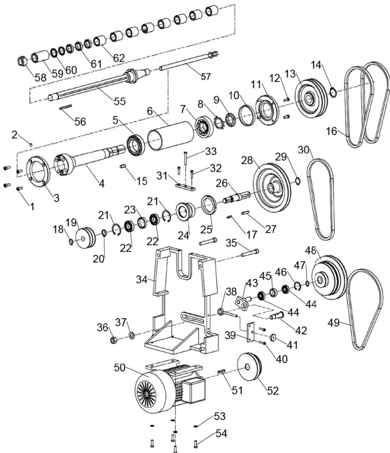
Abb.1-4: Riementrieb Horizontalfräsen - Belt drive horizontal milling
