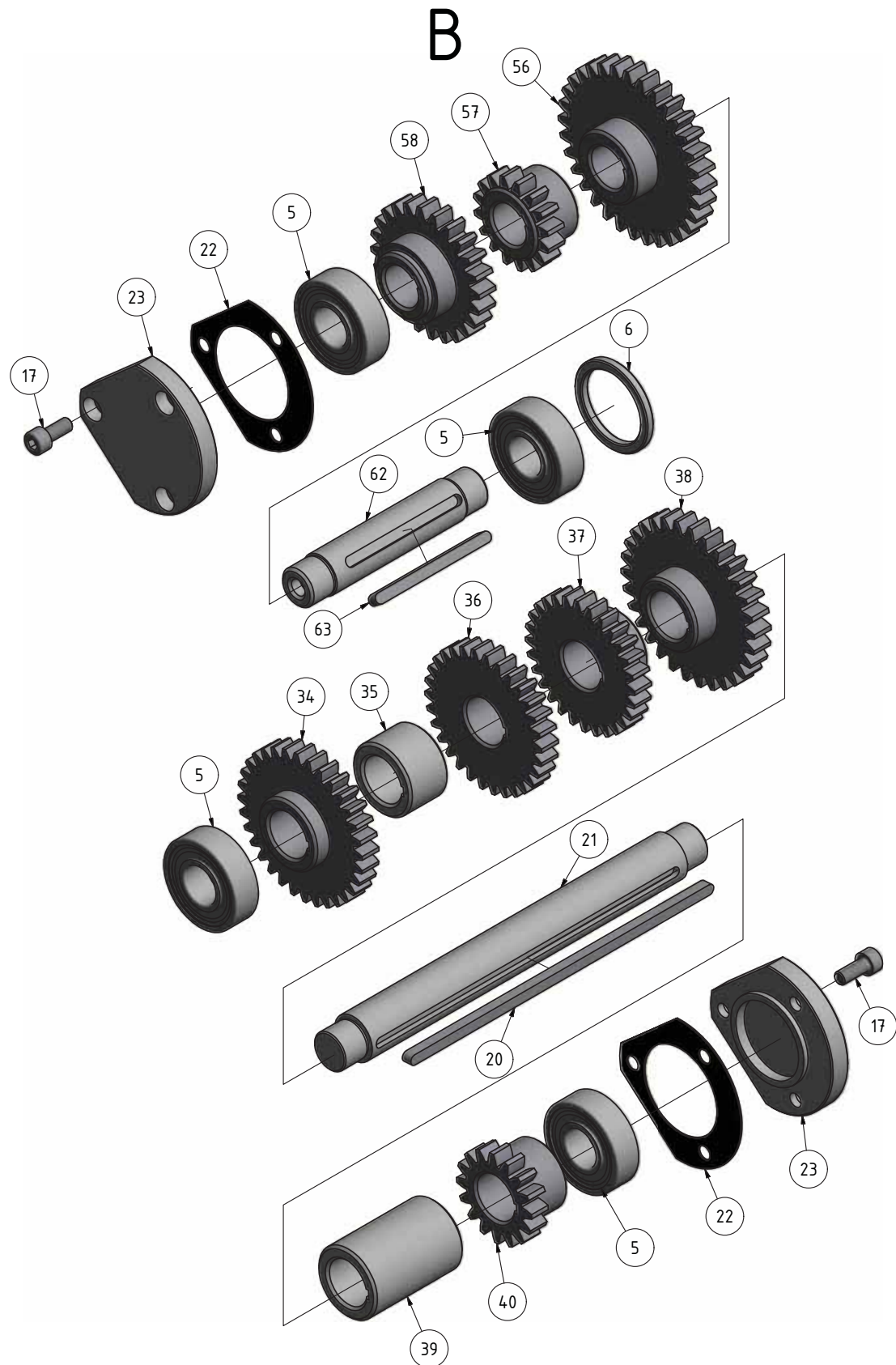
Img.1-13: Vorschubgetriebe 4-6 - Feed gear 4-6
