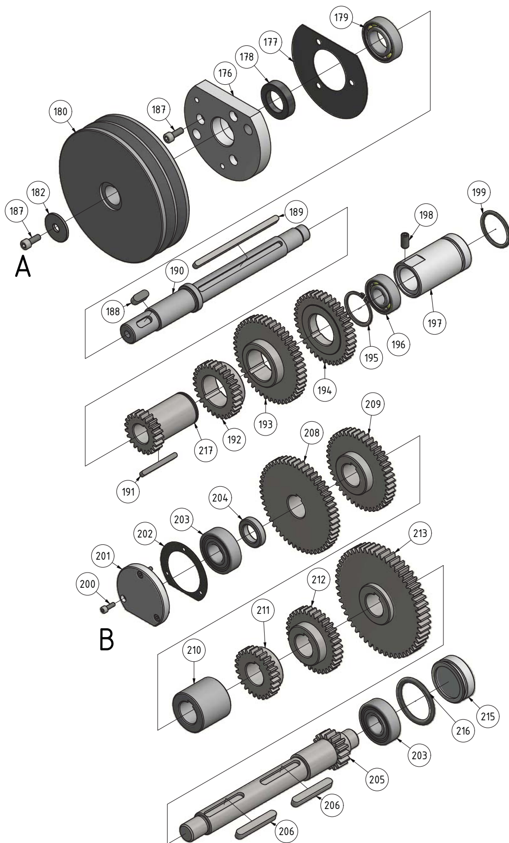
Img.1-6: Getriebe Spindelstock 3-6 - Headstock gear 3-6
