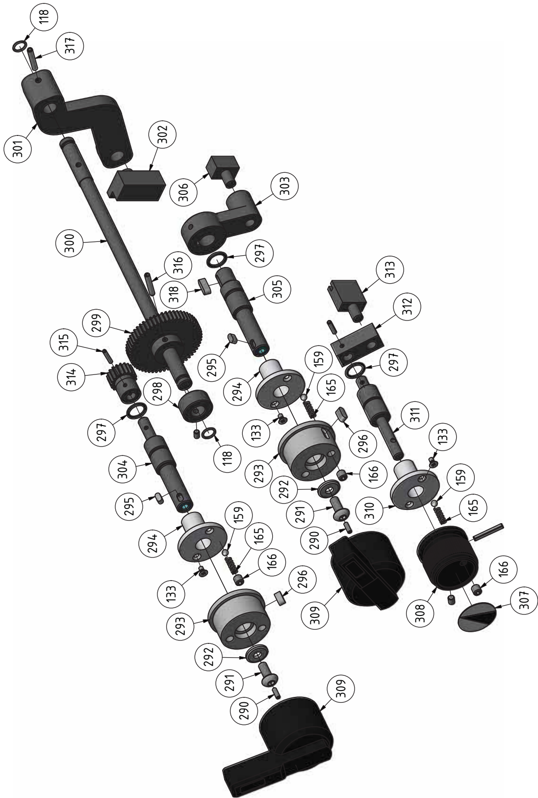
Img.1-9: Getriebe Spindelstock 6-6 - Headstock gear 6-6
