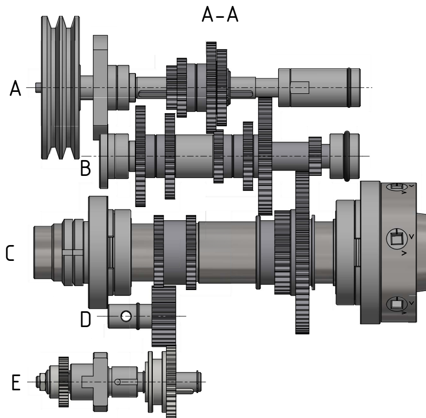
Img.1-5: Getriebe Spindelstock 2-6 - Headstock gear 2-6
