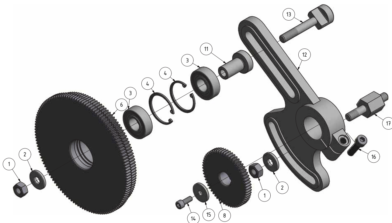
Img.1-16: Wechselradgetriebe- Change gear
