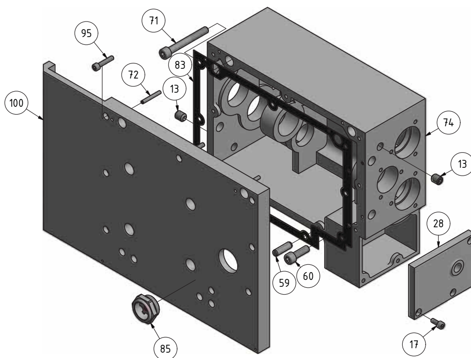
Img.1-10: Vorschubgetriebe 1-6 - Feed gear 1-6
