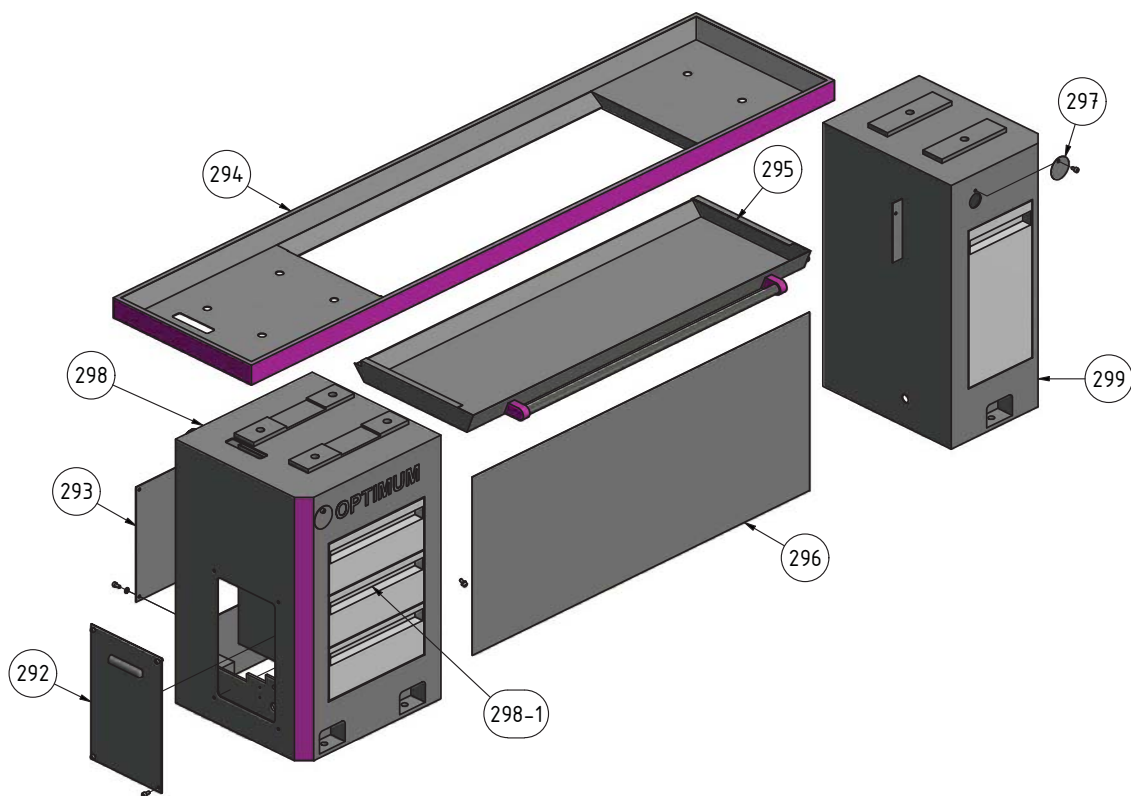
Img.1-2: Maschinenunterbau - Substructure
