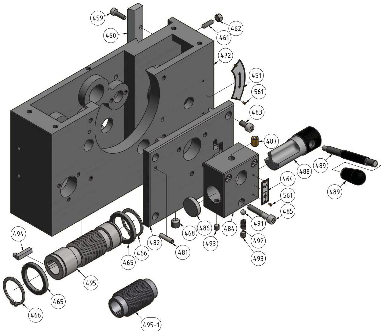
Img.1-17: Schlosskasten 1-3 - Apron 1-3
