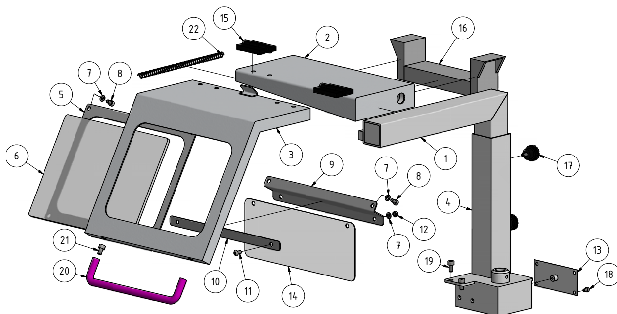
Img.1-26: Späneschutz - Chip protection
