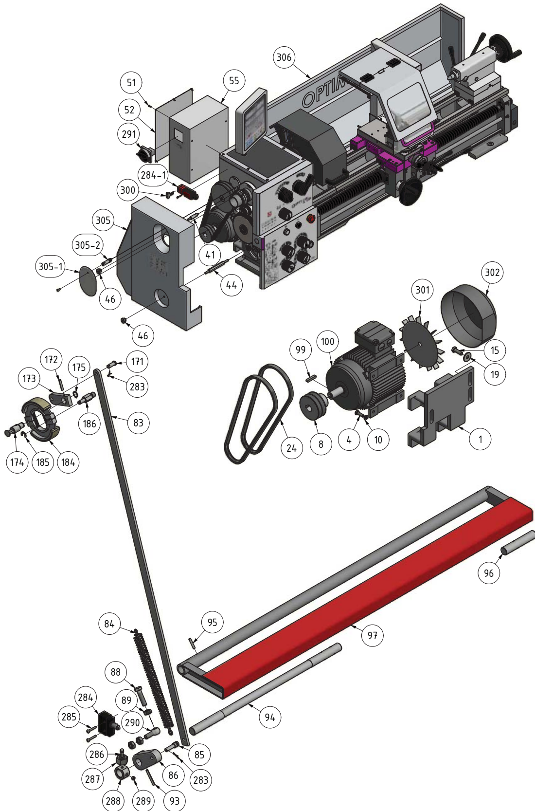
Img.1-1: Antrieb - Drive
