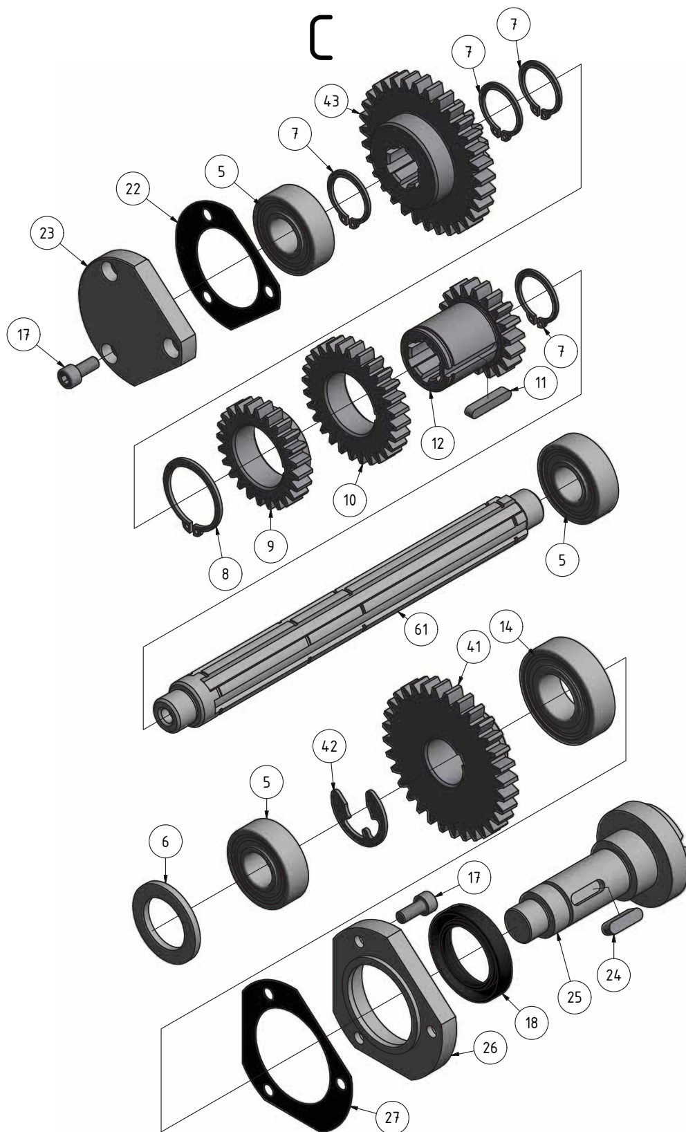
Img.1-14: Vorschubgetriebe 5-6 - Feed gear 5-6
