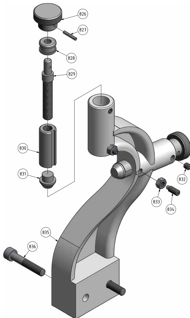
Img.1-24: Mitlaufende Lünette - Follow rest
