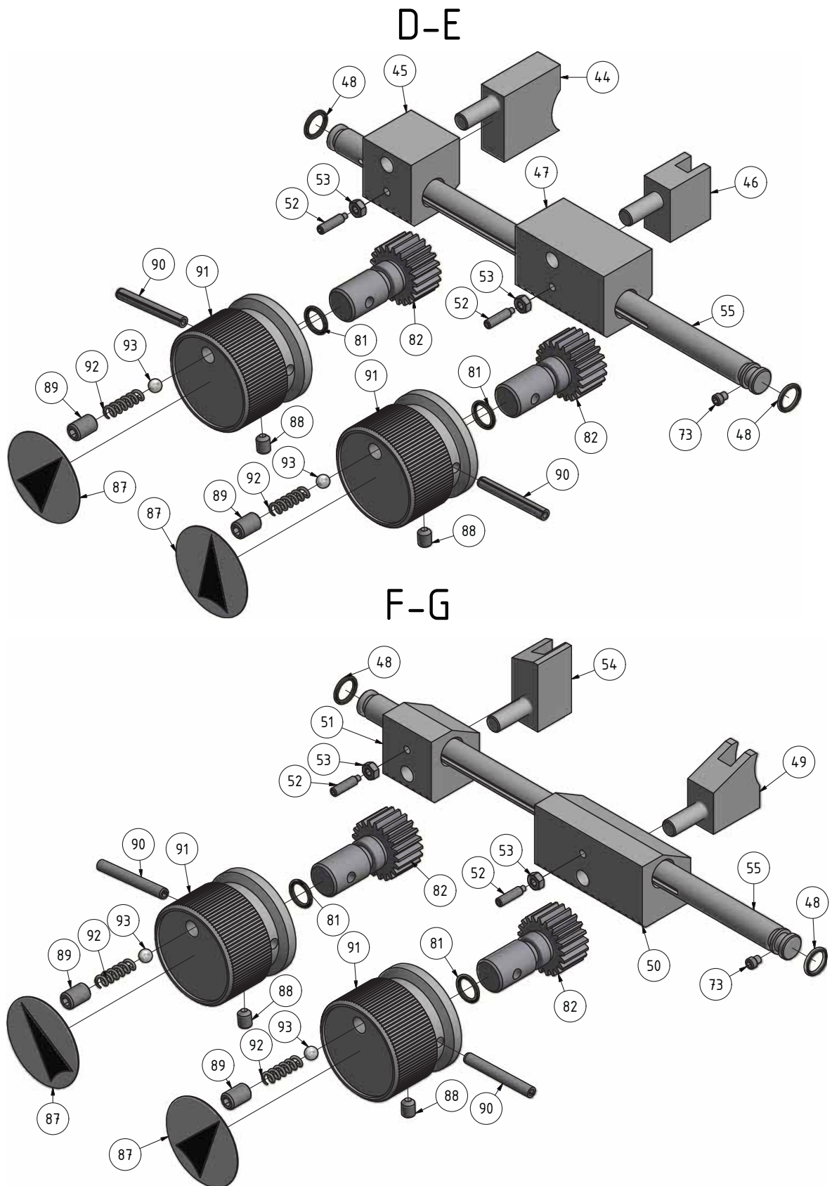
Img.1-15: Vorschubgetriebe 6-6 - Feed gear 6-6
