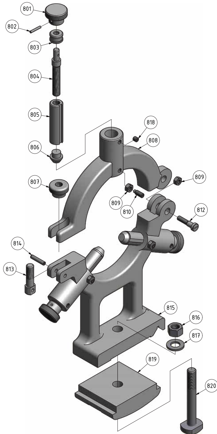
Img.1-23: Feststehende Lünette - Steady rest
