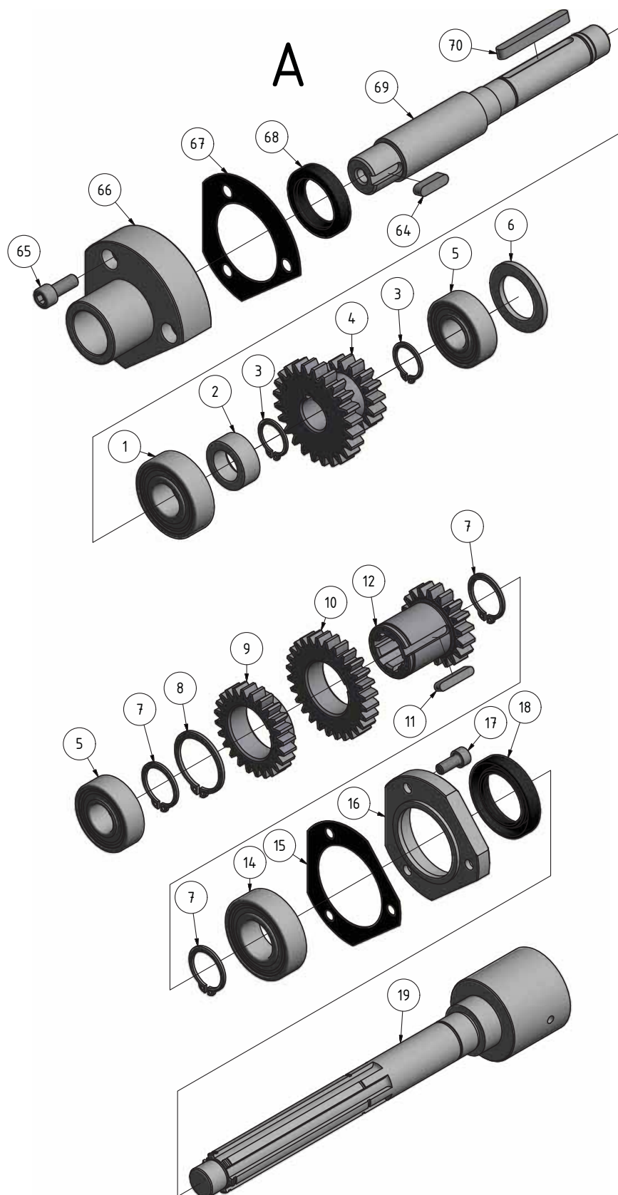
Img.1-12: Vorschubgetriebe 3-6 - Feed gear 3-6
