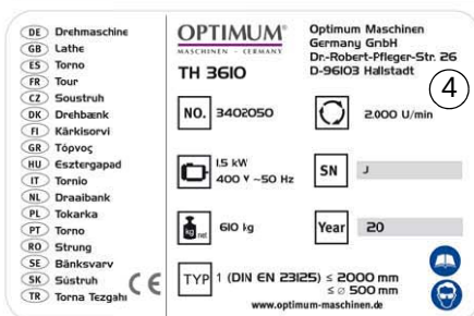
Img.1-27: Maschinenschilder - Machine labels
