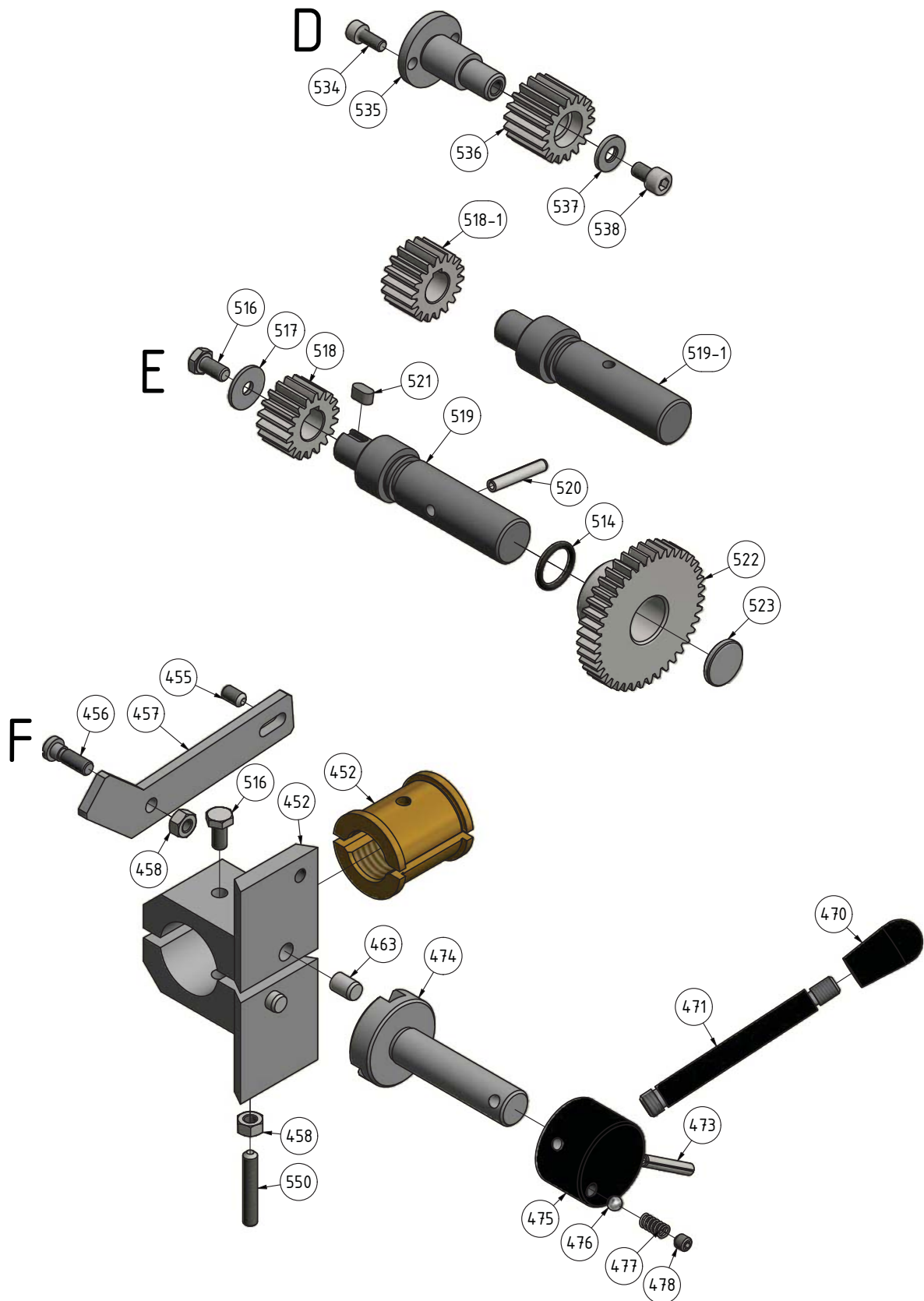
Img.1-19: Schlosskasten 3-3 - Apron 3-3
