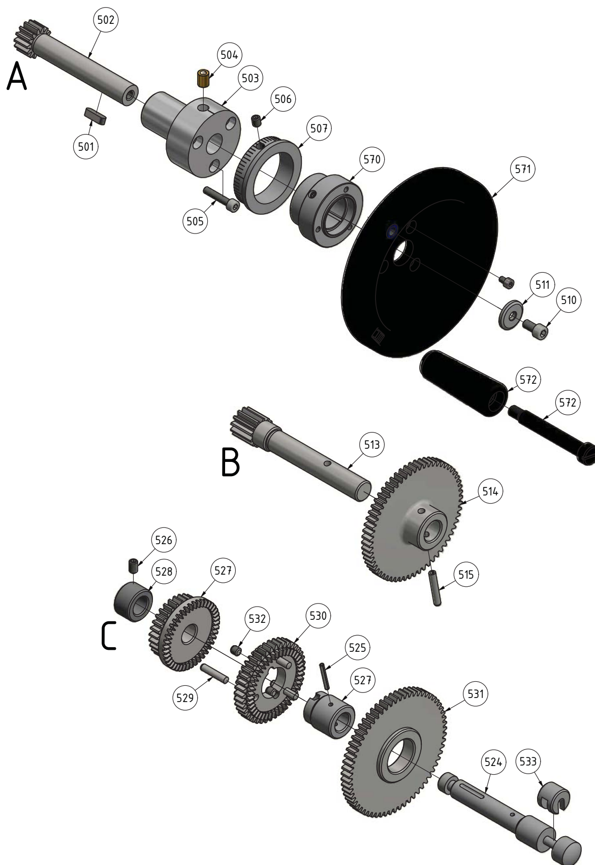
Img.1-18: Schlosskasten 2-3 - Apron 2-3
